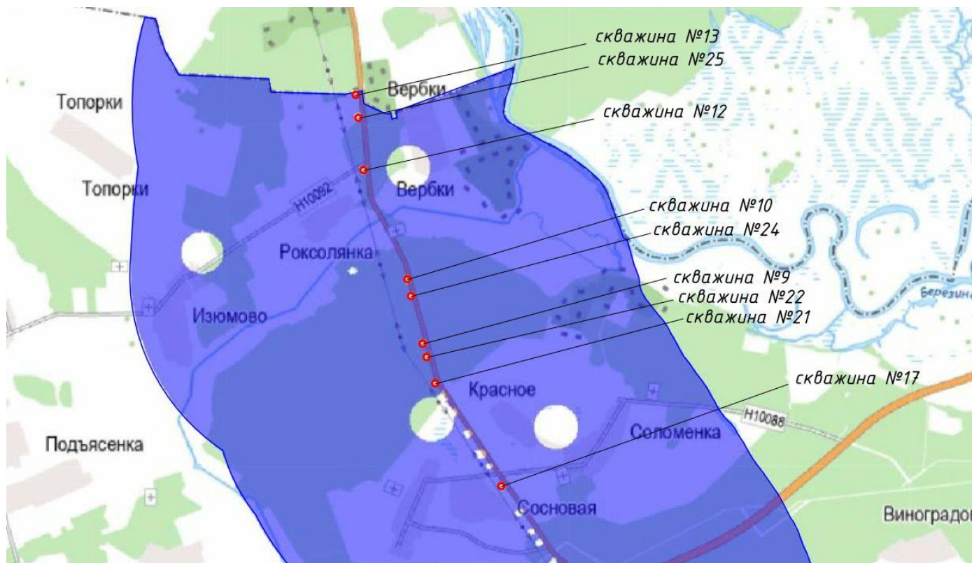
Рис. 2.1 – Месторасположение новых и тампонируемых существующих скважин водозабора № 4
